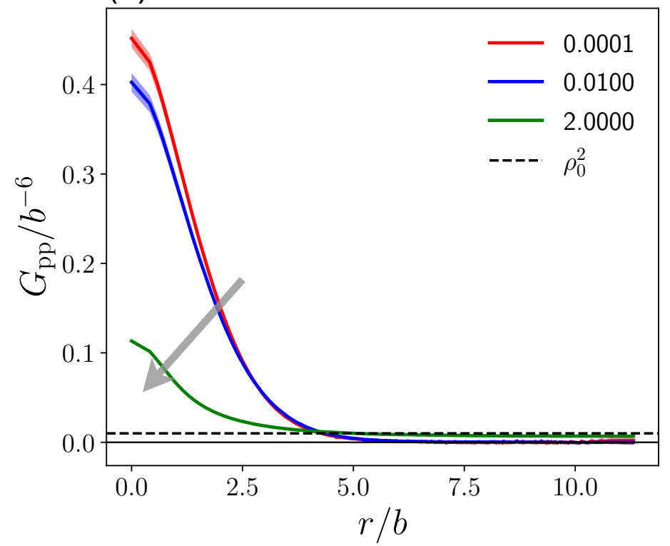
(d) [Na + ] = 10 -4 0.01 2.0
