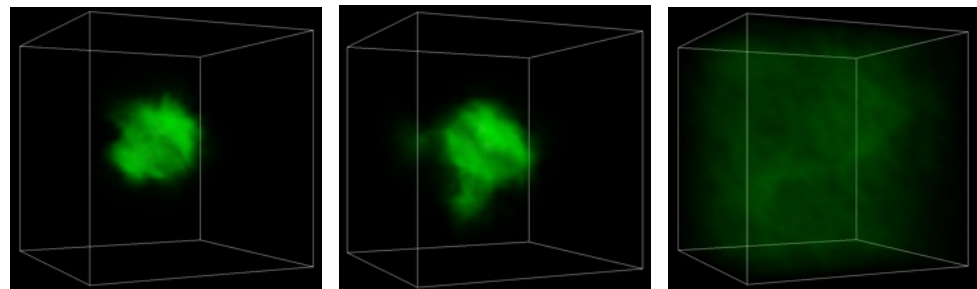
(d) [Na + ] = 10 -4 0.01 2.0
